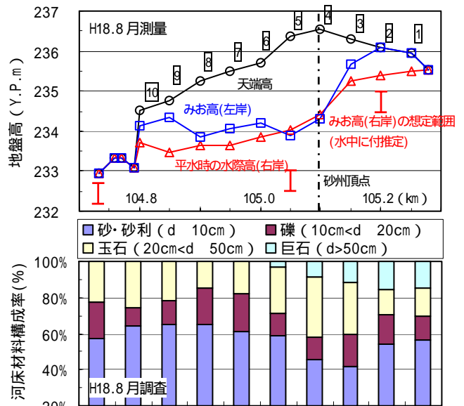
図-4 砂礫砂州の縦断形状と河床材料
