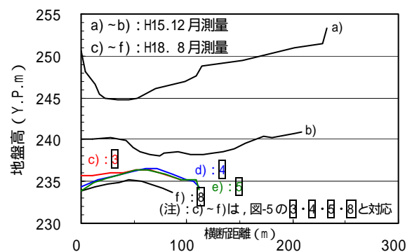
図-3 横断形状(小林橋上流地区(104.5k~107k))
