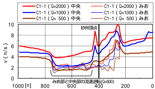
図-9 CASE1-1 における河道中央・みお筋の縦断流速分布
