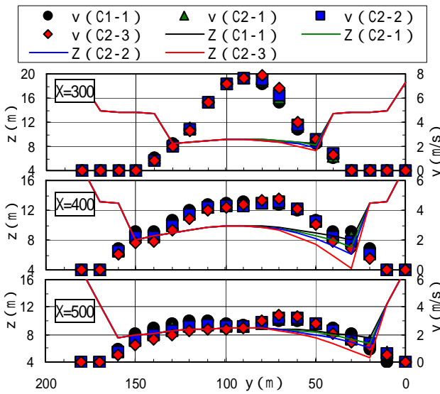
図-13 Q=1000m^3/s におけるCASE別の横断流速分布
