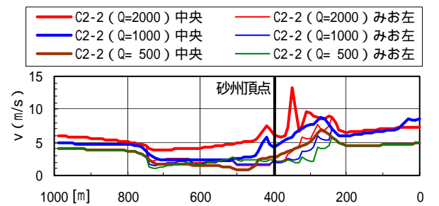
図-15 CASE2-2における河道中央・みお(左)の縦断流速分布
