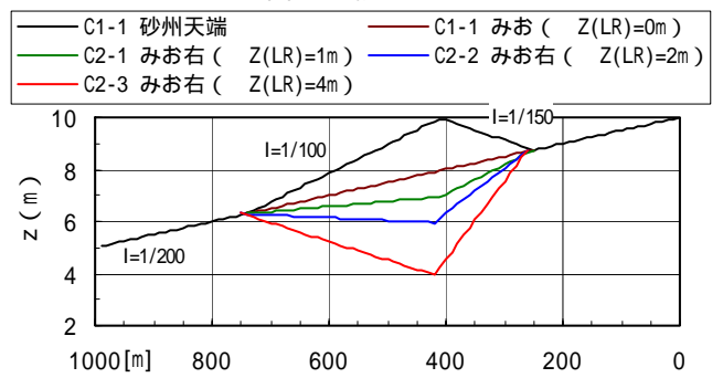
図-8 砂州天端とみお筋の縦断形状
