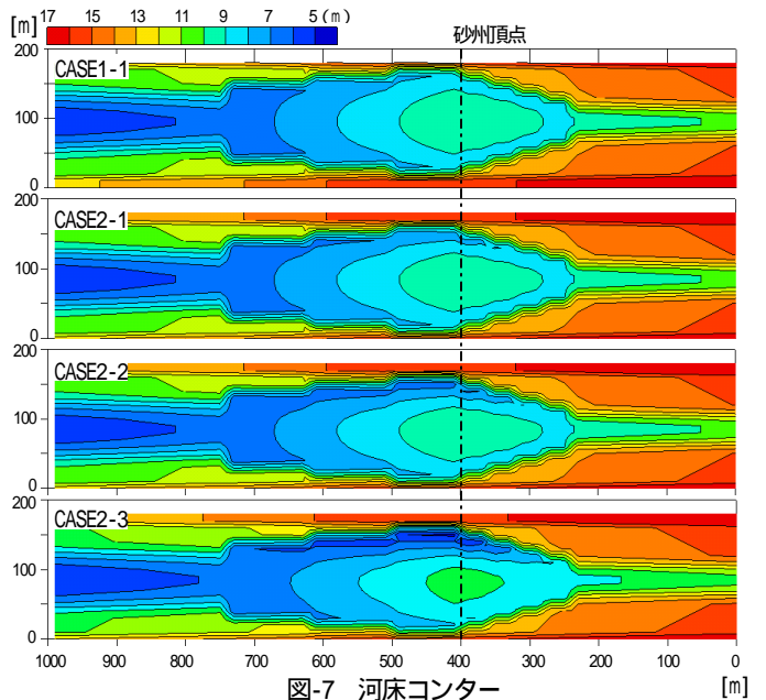
図-7 河床コンター
