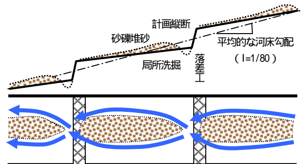
図-2 流路工施工に伴う流路変化の模式図
