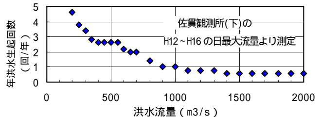
図-6 年間の洪水発生回数(佐貫観測所(下))
