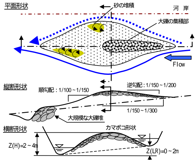
図-1 砂礫砂州の基本構造の模式図
