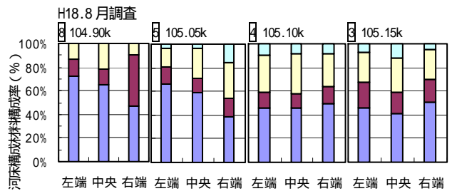
図-5 砂礫砂州の横断方向の河床材料(③・④・⑤・⑧)
