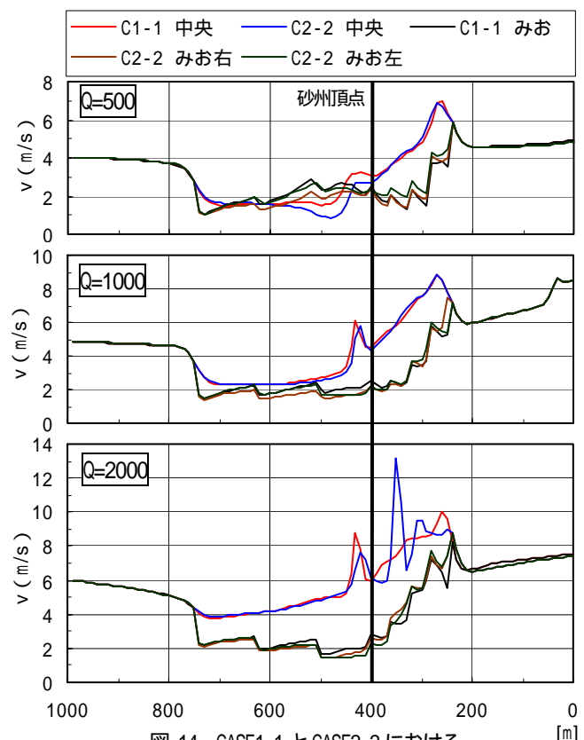
図-14 CASE1-1とCASE2-2における流量別の河道中央・みお筋の縦断流速分布
